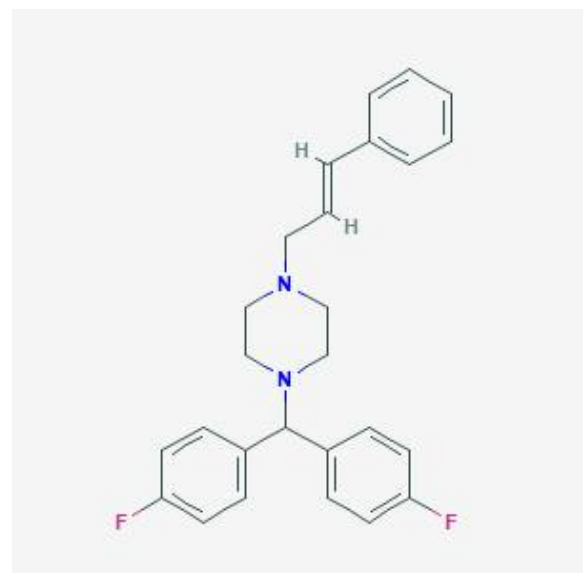
그림 1. 플루나리진의 구조식
